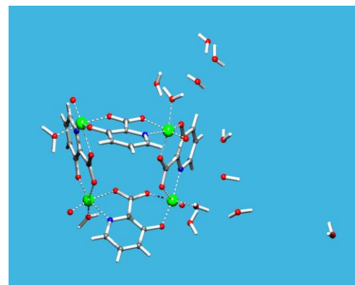
Vanadil komplex
