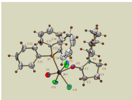
Rénium komplex
